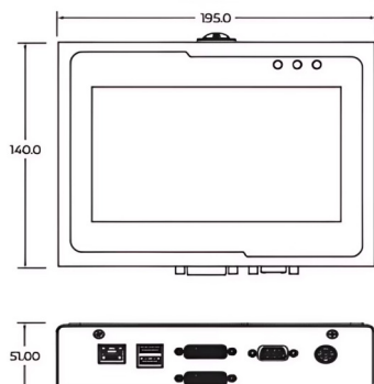
R20e Controller — 195.0mm (W) × 140.0mm (H) × 51.00mm (D)
